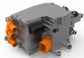
3 in1 unit: 22kW OBC, 3,7kW DCDC, ECU
